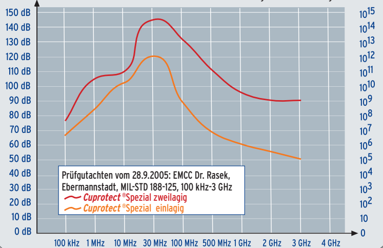
Cuprotect ® Spezial Schirmdämpfung in dB
